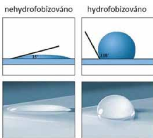
Obr. 1 - Smáčecí úhel
