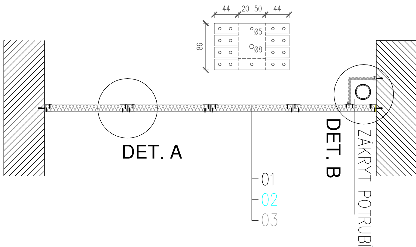
KONSTRUKČNÍ SPOJKA
