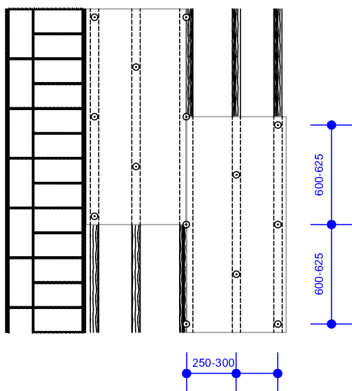
SCHÉMA MONTÁŽNÍ KONSTRUKCE
