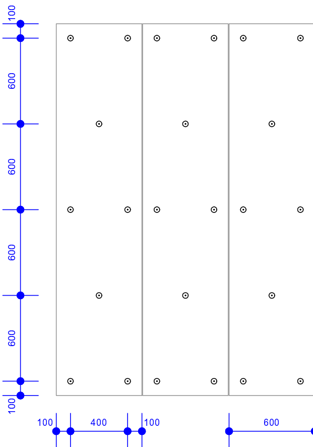
Celoplošné (bodové) lepení a kotvení pro KONSTRUKČNÍ DESKY o tloušťce 30, 40 a 50 mm.
