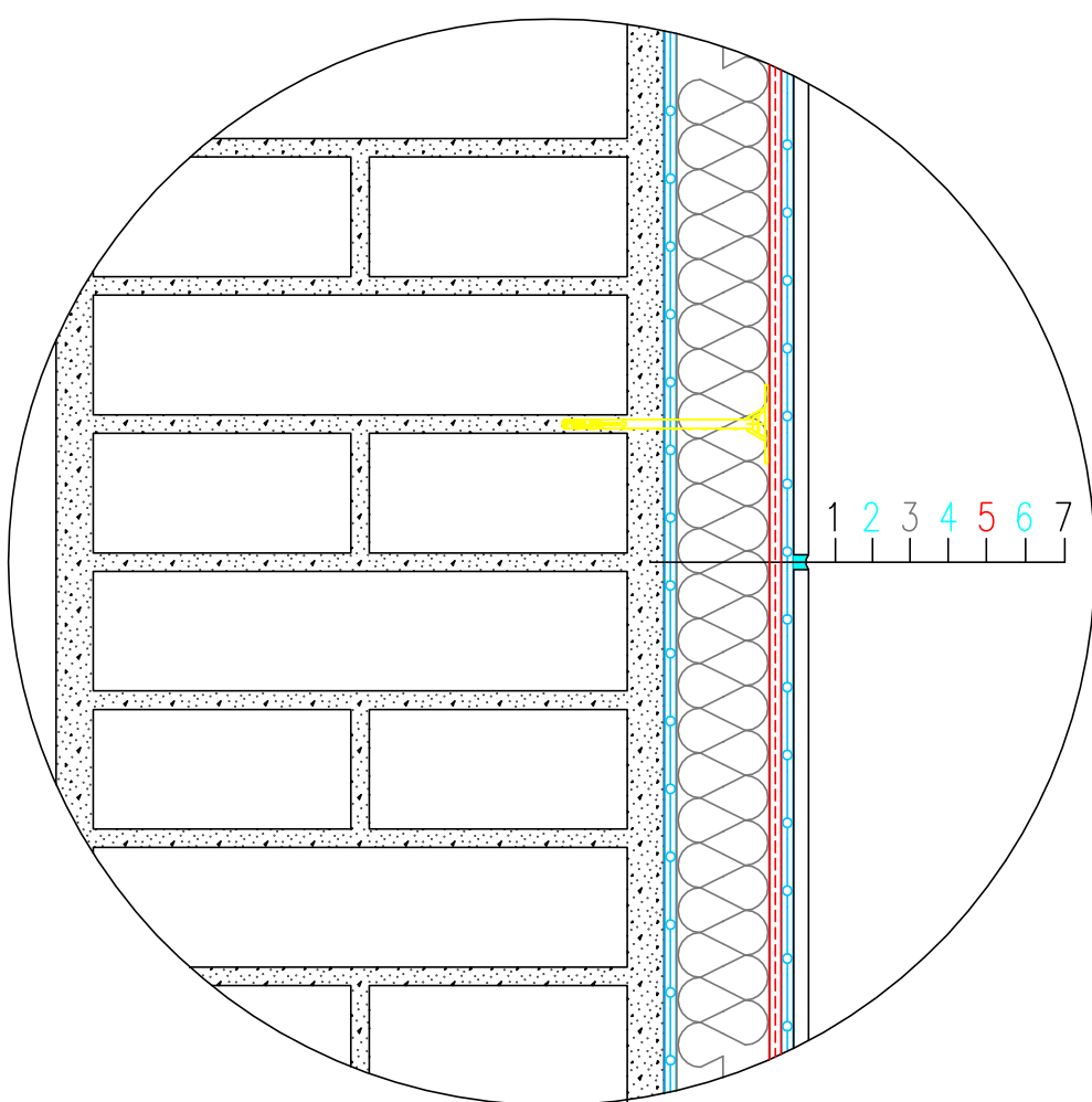
Celoplošné lepení a kotvení pro KONSTRUKČNÍ DESKY o tloušťce 6, 10 a 20 mm.
